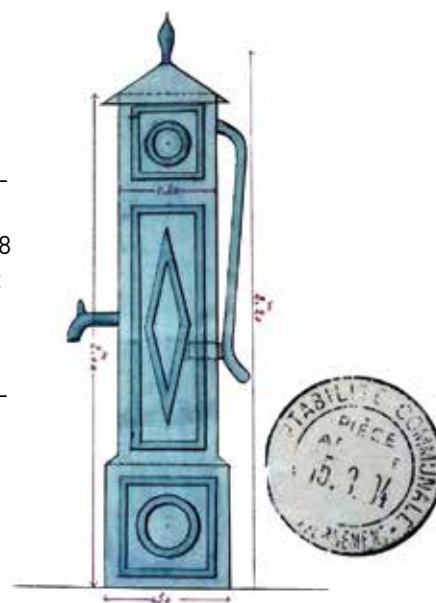
Der Plan eines Brunnenkastens aus dem Jahre 1898 (Archiv der Stadt Ettelbrück)
